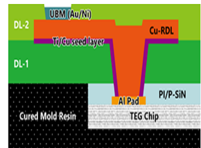
FOWLP 断面図
